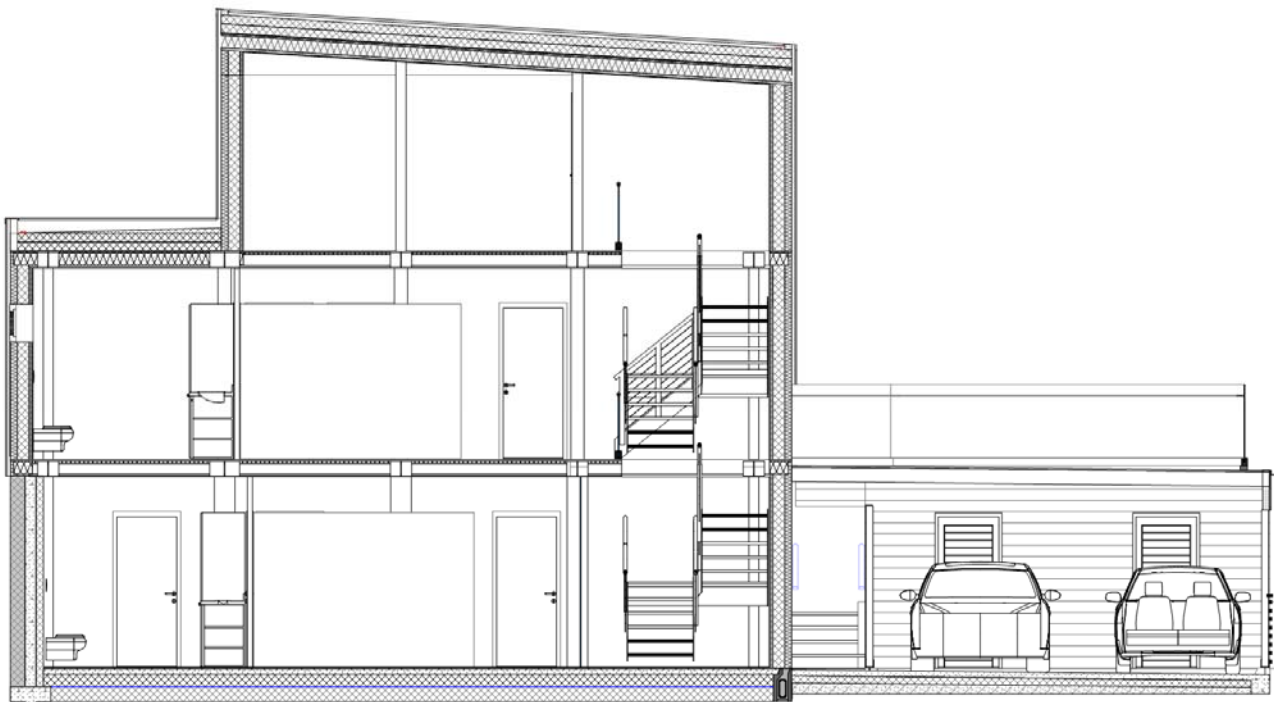
Snitt B
